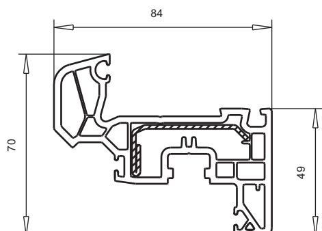
арт. № 103.313 пленка с двух сторон пленка с одной стороны усилитель арт. №113.269
