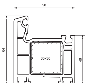
арт. № 101.213 пленка с двух сторон пленка с одной стороны усилитель арт. № 113.025
