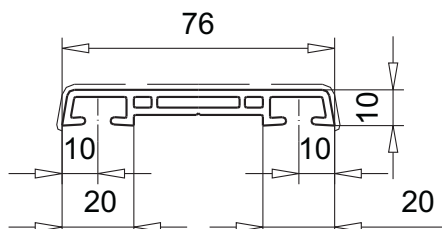
облицовочный профиль арт.№ 109.208 клеммниппель арт.№ 108.016
