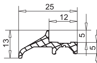
алюминиевый слезник 25/12мм
