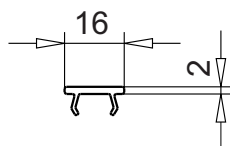
заполняющий профиль арт.№ 109.045 для фурнитурного паза Цвет: белый, коричневый
