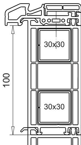
профиль для уплотнения из ПВХ арт. № 104.128 Цвет: черный / с клеящей лентой / с отверстиями уплотнитель арт. № 112.026
