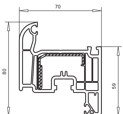
арт. № 103.235 пленка с двух сторон пленка с одной стороны усилитель арт. №113.292 усилитель арт. №113.294 усилитель арт. №113.295
