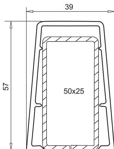
внешний усилитель 39x57 мм
