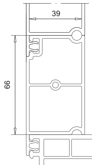
коробка 66x39 мм арт. № 109.356
