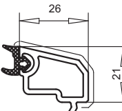
арт. №107.207 контур TOPLINE
