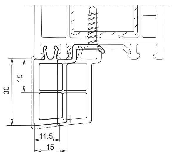
профиль для присоединения отлива арт. № 110.047
