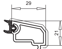
арт. №107.206 контур TOPLINE
