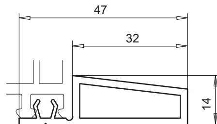
маскирующий профиль арт. № 109.231
