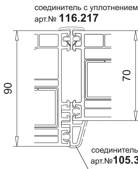
арт.№ 105.316.2 соединитель вертикальный
