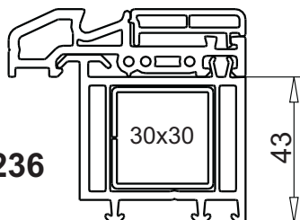
арт. № 109.445 усилитель 113.025 (на выбор)
