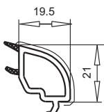
арт. №107.236 контур SWINGLINE
