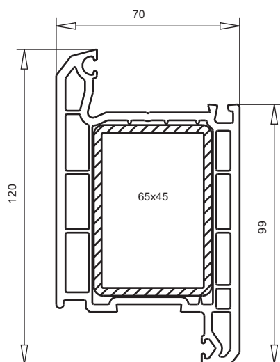
арт. № 105.200 дверная створка пленка с двух сторон пленка с одной стороны усилитель арт. № 113.286.3 алюмин.усилитель арт.№ 115.200
