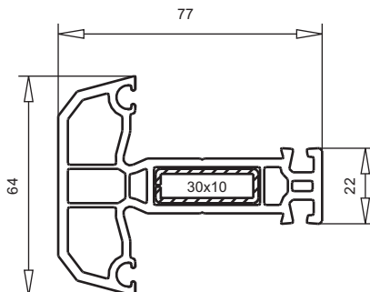
арт. № 102.209 створочная перекладина пленка с двух сторон пленка с одной стороны усилитель арт. №113.020
