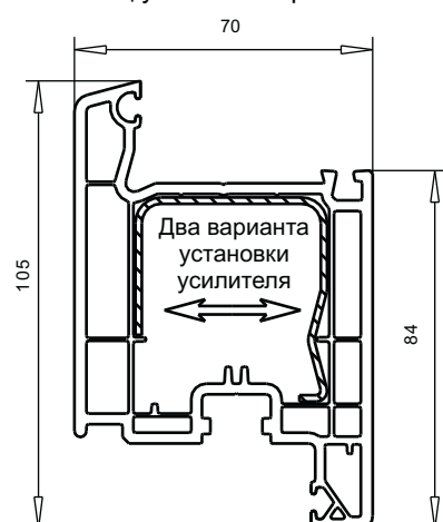
арт. № 103.241
