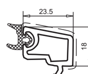
штапик арт. № 107.583
