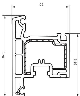
арт. № 103.213 усилитель арт. № 113.229
