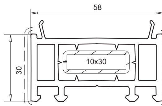
расширитель 30 мм арт. № 114.012 усилитель арт. № 113.020
