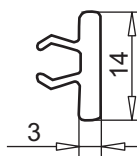
заглушка из ПВХ арт. № 109.037 для порога 104.037 цвет: белый, коричневый
