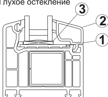
Глухое остекление
