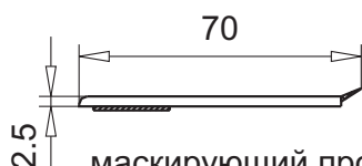
маскирующий профиль 70мм арт.№ 109.441.3 с резинкой, белый с клеящейся лентой 19х1мм, черный
