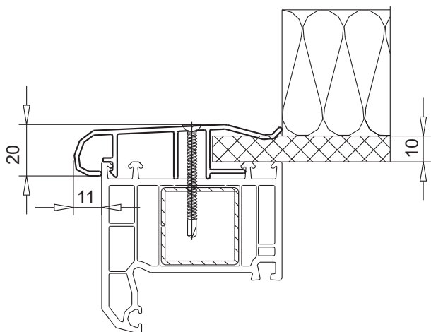
скругляющий профиль 20мм для 10мм плиты арт.№ 108.077
