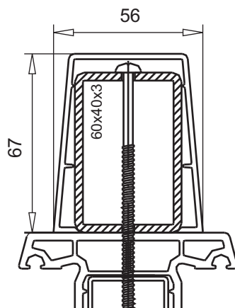
внешний усилитель арт.№ 114.019 усилитель 60x40x2.0 арт.№ 113.011.2 I_x=10.23\text{см}^4 ; I_y=19.31\text{см}^4 усилитель 60x40x3.0 арт.№ 113.011.3 I_x=14.32\text{см}^4 ; I_y=27.39\text{см}^4
