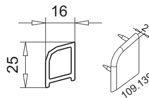
защитная планка арт.№ 109.112 заглушка арт.№ 109.139 Цвет: белый
