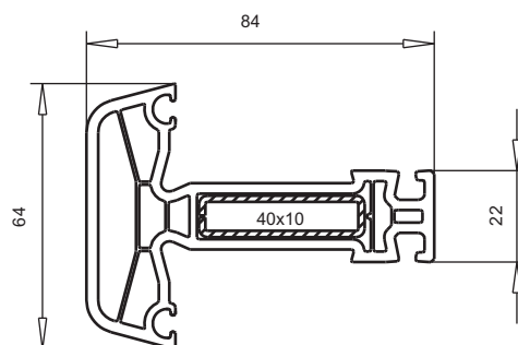
арт. № 102.243 створочная перекладина пленка с двух сторон пленка с одной стороны усилитель арт. №113.028
