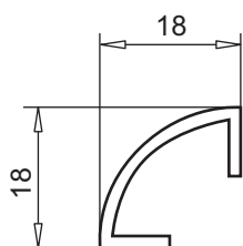
закрывающая планка арт. № 117.857
