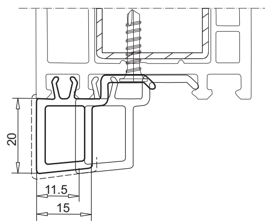
профиль для присоединения отлива арт. № 110.048
