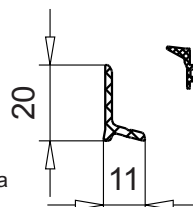
алюм.уголок (для противовзломного окна) арт.№ 104.209 Цвет: алюм.красный уплотнение арт.№ 112.261 АРТК серый
