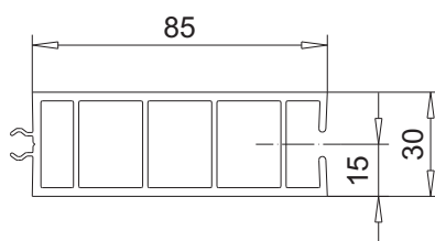
вставка арт. № 109.210
