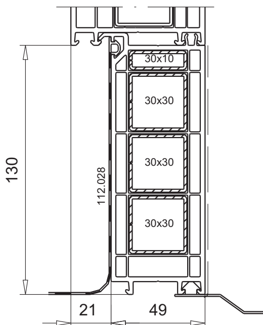
расширительный профиль для балконной двери арт.№ 109.569 усилитель арт.№ 113.025 / 113.020 специальная анкерная пластина арт.№ 141.137
