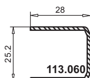
арт. № 101.287 усилитель арт. № 113.002 усилитель арт. № 113.060
