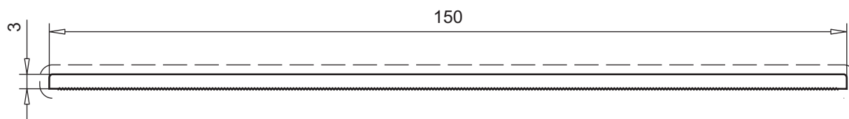
полоса 150 мм арт. № 109.054
