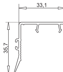
арт. № 105.372 закрывающая планка
