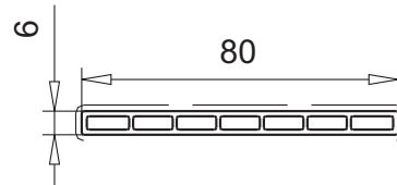
облицовочный однокамерный профиль 80мм 109.046
