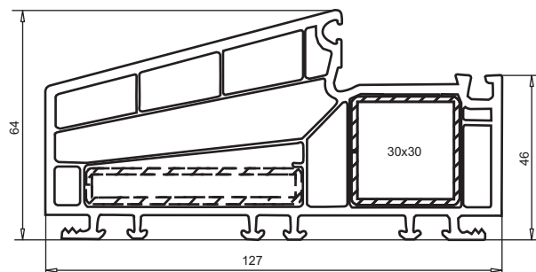
арт. № 101.151 усилитель арт. № 113.025
