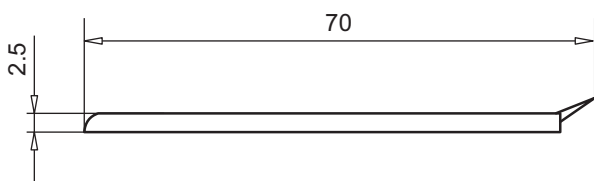
маскирующий профиль 20 мм арт. № 109.442.2
