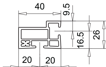
присоединительный профиль арт.№ 109.073 клеммниппель арт.№ 108.016
