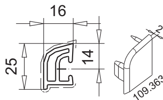
защитная планка арт.№ 109.346 заглушка арт.№ 109.363 Цвет: белый, коричневый, охра, черный клеммниппель арт.№ 108.016
