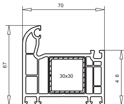
арт. № 101.233 пленка с двух сторон пленка с одной стороны усилитель арт. №113.025
