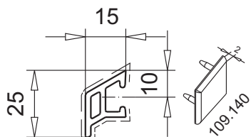
защитная планка арт.№ 109.030 заглушка арт.№ 109.140 Цвет: белый, коричневый клеммниппель арт.№ 108.016
