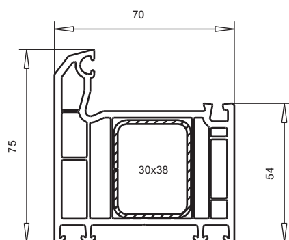
арт. № 101.205 пленка с двух сторон пленка с одной стороны усилитель арт. № 113.271 усилитель арт. № 113.302
