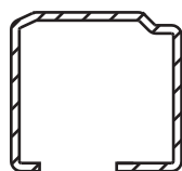
арт. № 113.049.2 усилитель
