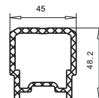
алюмин. усилитель (только для белых профилей) арт. № 115.003
