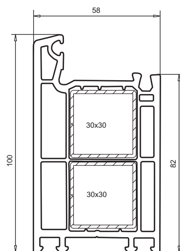
арт. № 101.094 пленка с двух сторон пленка с одной стороны усилитель арт. № 113.025 /2 шт.
