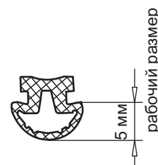
дверное уплотнение арт. № 112.026 цвет: черный
