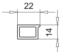
профиль арт.№ 109.097
