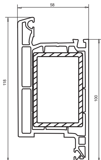
арт. № 105.123 дверная створка пленка с двух сторон пленка с одной стороны усилитель арт. № 113.011.3
