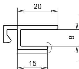
стыкующий профиль арт. № 109.286
