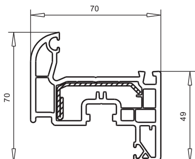
арт. № 103.272 пленка с двух сторон пленка с одной стороны усилитель арт. №113.269
