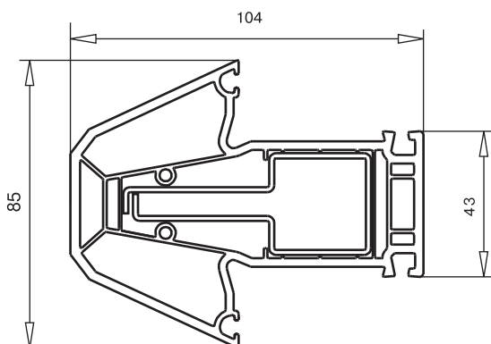
арт. № 102.230 ИМПОСТ усилитель арт. №113.025/113.329/ 113.329.2/113.343.2
