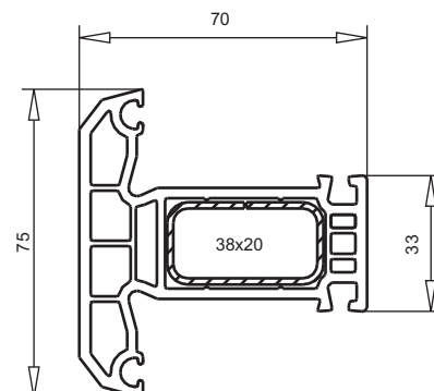
арт. № 102.201 пленка с двух сторон пленка с одной стороны усилитель арт. №113.272
