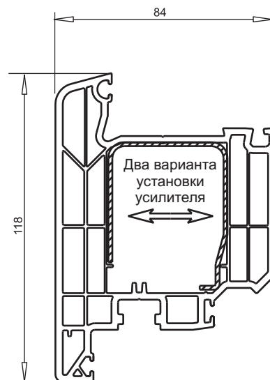
арт. № 103.330 , наружное открывание пленка с двух сторон пленка с одной стороны усилитель арт. №113.304
