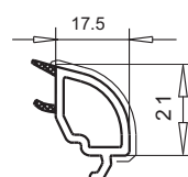
арт. №107.237 контур SWINGLINE
