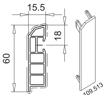
облицовочный профиль арт.№ 109.205 заглушка арт.№ 109.513 Цвет: белый клеммниппель арт.№ 108.016
