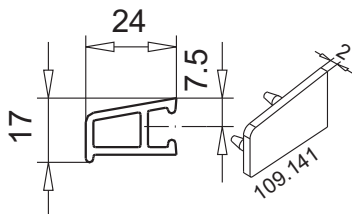
защитная планка арт.№ 109.122 заглушка арт.№ 109.141 Цвет: белый клеммниппель арт.№ 108.016
