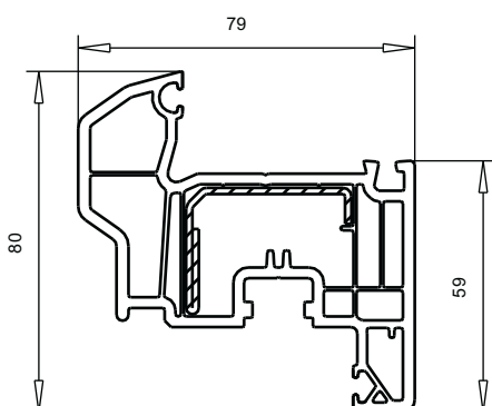
арт. № 103.238
