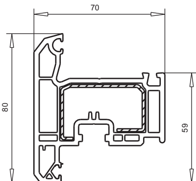
арт. № 103.205 наружное открывание пленка с двух сторон усилитель арт. №113.276
