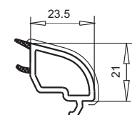
арт. №107.235 контур SWINGLINE
