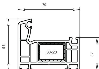
арт. № 101.207 пленка с двух сторон пленка с одной стороны усилитель арт. № 113.019
