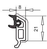
арт. №107.225 контур SOFTLINE
