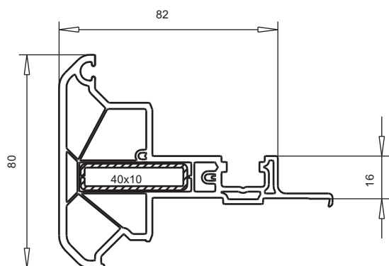
арт. № 102.244 пленка с двух сторон пленка с одной стороны усилитель арт. №113.028
