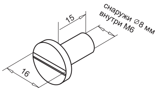
гильза для SL AD арт. № 141.124.2 никелированная латунь
