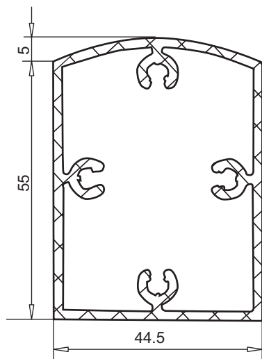
порог для входной двери арт. № 104.009 цвет: алюмин., E6/EV1, Euras 15
