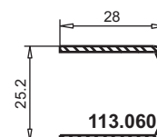
арт. № 103.329 усилитель арт. № 113.229 усилитель арт. № 113.060
