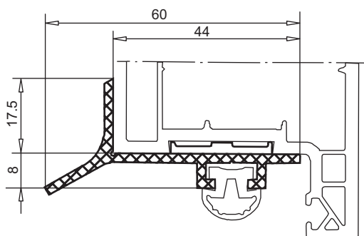
профиль с пазом под уплотнение арт. № 104.011 цвет: белый, коричневый
