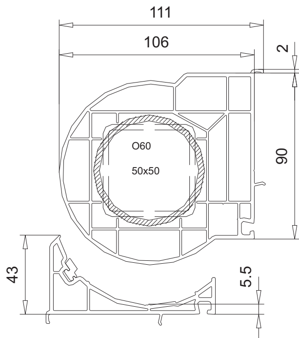
присоединительный профиль арт.№ 116.215 уплотнение 112.253
