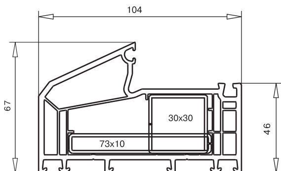
арт. № 101.230 усилитель арт. №113.271/113.330/113.342
