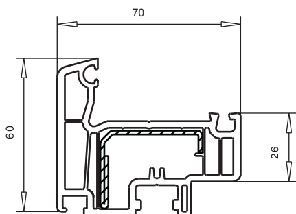
арт. № 103.293 усилитель арт. №113.292/113.294 заглушка арт. №109.566 (16,5 мм) заглушка арт. №109.562 (18,5 мм)
