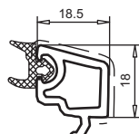
штапик арт. № 107.591
