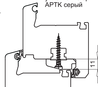
водоотводная трубка арт. № 143.062 прозрачная внешний \varnothing 10\text{мм} / общая длина 11.5мм
