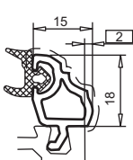
штапик арт. № 107.595
