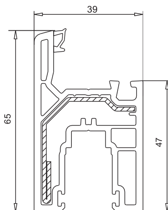
арт. № 105.371 створка усилитель арт. №113.056
