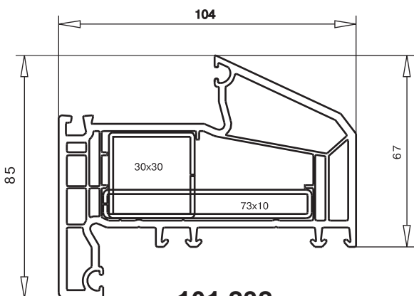
арт. № 101.232 усилитель арт. №113.025/113.330/113.342
