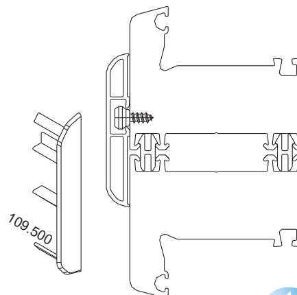
облицовочный профиль арт.№ 109.499 заглушка арт.№ 109.500 Цвет: белый клеммниппель арт.№ 108.016
