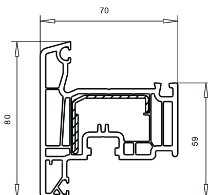
арт. № 103.228
