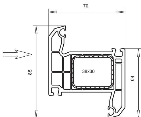
переходной профиль
