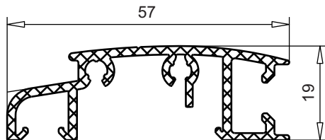
порог для входной двери арт. № 104.422 цвет: алюминий, серебристый, Euros
