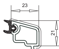
арт. №107.210 контур SOFTLINE
