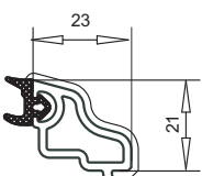
арт. №107.211 контур SOFTLINE
