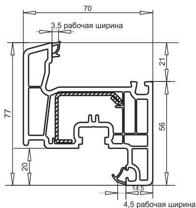
арт. № 103.323 усилитель арт. № 113.010
