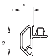
арт. № 109.560 упорная планка заглушка арт. №109.567
