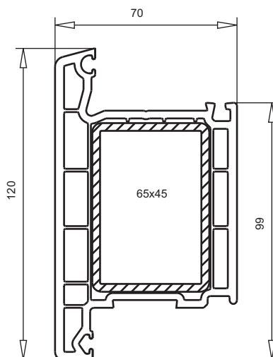
арт. № 105.233 дверная створка наружного открывания пленка с двух сторон пленка с одной стороны усилитель арт. № 113.286.3 алюмин.усилитель арт. № 115.200
