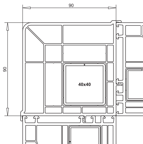
соединитель угловой 90° арт.№ 116.214 усилитель 113.281.2
