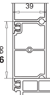
облицовочный профиль арт.№ 109.231 клипсовое соединение на раму
