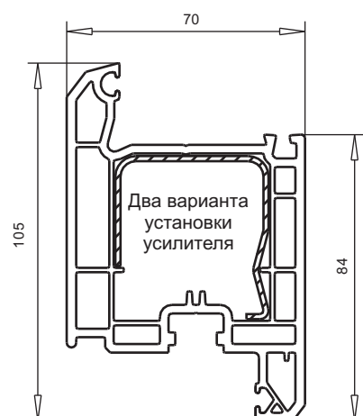
арт. № 103.202 пленка с двух сторон пленка с одной стороны усилитель арт. №113.270 алюмин.усилитель арт.№115.003 (только для белых профилей)
