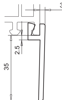
маскирующий профиль арт. № 109.402
