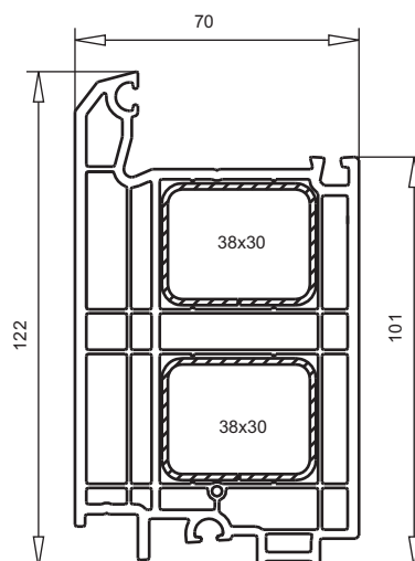
арт. № 105.202 пленка с двух сторон пленка с одной стороны усилитель арт. № 113.271 уплотнение арт.№ 112.253 импостной соединитель с уплотнительной пластиной (разрезать на две половины) напр.арт.№116.200.1
