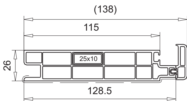
рамный профиль арт.№ 109.582
