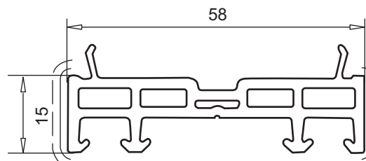
расширитель 15 мм арт. № 114.024
