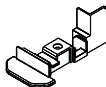
Заглушка арт. № 109.519 Цвет: белый, черный, охра
