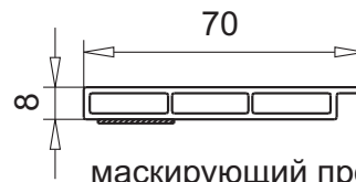
маскирующий профиль 70мм арт.№ 109.444.3 с клеящейся лентой 19х1мм, черный
