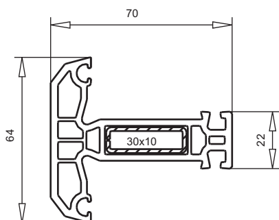
арт. № 102.208 створочная перекладина пленка с двух сторон пленка с одной стороны усилитель арт. №113.020
