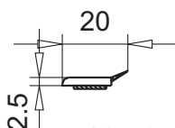
маскирующий профиль 20мм арт.№ 109.438.3 с резинкой, белый с клеящейся лентой, 10х1мм, черный
