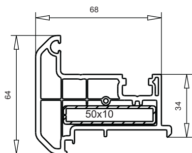
арт. № 102.236 пленка с двух сторон пленка с одной стороны усилитель арт. № 113.013 усилитель арт. № 113.013.3 (стальная полоска)
