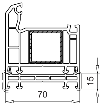
расширитель 15мм арт.№ 114.200/028
