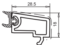
штапик арт. № 107.592
