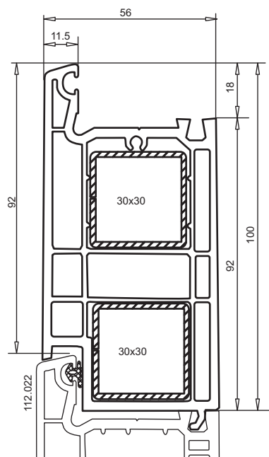
арт. № 105.083 расширительный профиль усилитель арт. № 113.025 уплотнение арт. № 112.022
