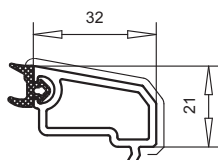
арт. №107.205 контур TOPLINE
