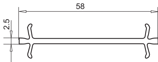
соединитель узкий арт. № 116.010 цвет: белый, коричневый
