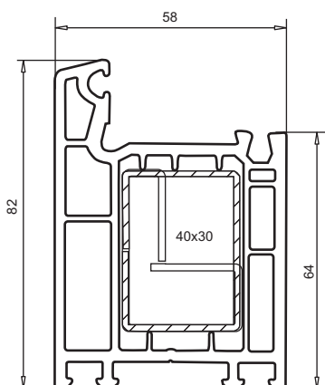
арт. № 101.085 пленка с двух сторон пленка с одной стороны усилитель арт. № 113.001 усилитель для входной двери арт. № 113.009
