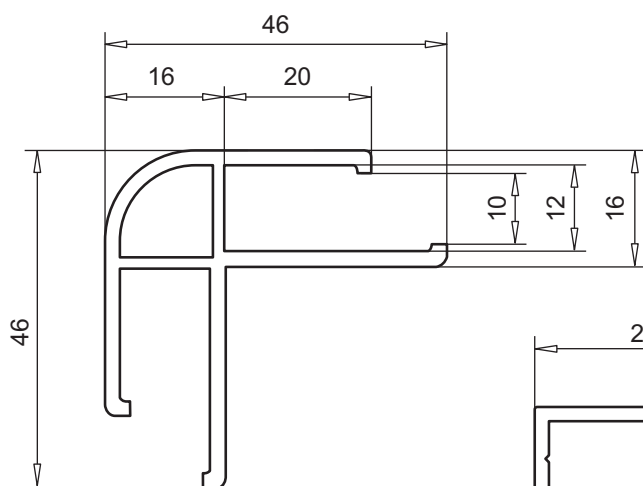
уголок 46 мм арт. № 109.406
