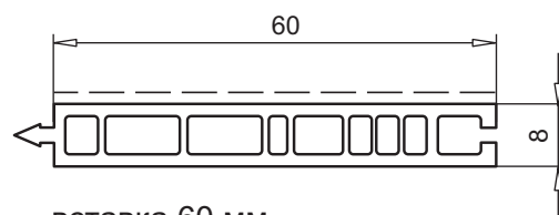
вставка 60 мм арт. № 119.024
