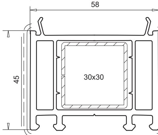
расширитель 30 мм арт. № 114.012 усилитель арт. № 113.020
