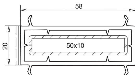
соединительный профиль арт. № 116.003 усилитель арт. №113.013 I_x=0,28 \text{ см}^4 , I_y=4,36 \text{ см}^4 стальная полоса арт. № 113.013.3 I_x=0,42 \text{ см}^4 , I_y=10,42 \text{ см}^4
