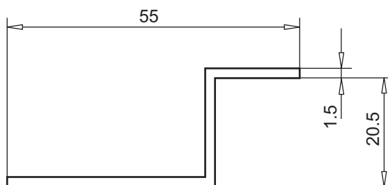
Z-образный профиль арт. № 117.834
