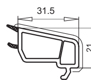
арт. №107.212 контур SOFTLINE
