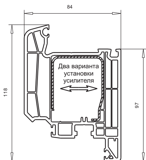
арт. № 103.314 пленка с двух сторон пленка с одной стороны усилитель арт. №113.304
