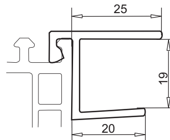
профиль с пазом арт. № 109.342
