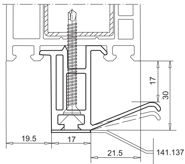
профиль для присоединения подоконника арт. № 110.054 для подоконника 17-22 мм анкер с захватом 141.137
