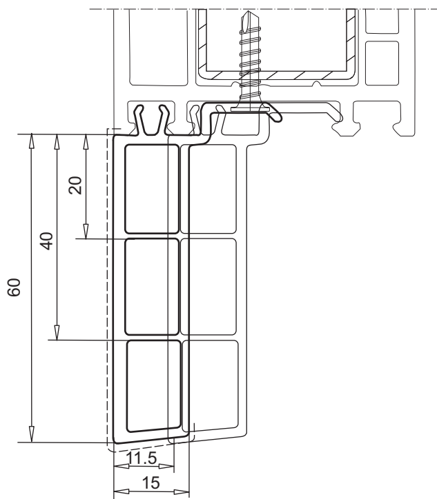
профиль для присоединения отлива арт. № 110.101
