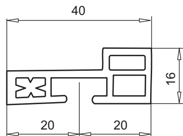
присоединительный профиль арт. № 109.072
