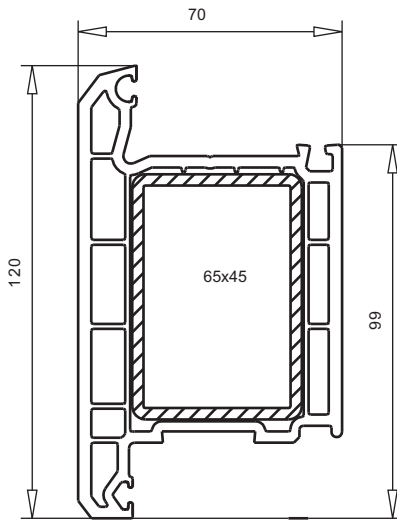
арт. № 105.210 дверная створка наружное открывание пленка с двух сторон пленка с одной стороны усилитель арт. № 113.286.3 алюмин.усилитель арт.№ 115.200
