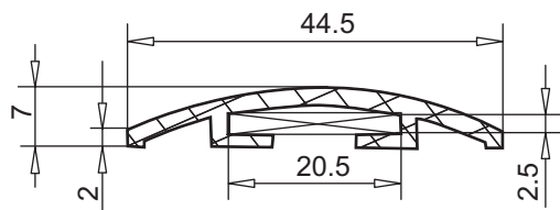
порог для входной двери крепится на шурупах арт. № 104.020 соединительный уголок 141.400.7 цвет: алюминий, E6/EV1
