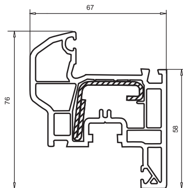
арт. № 103.274 полусовмещенная усилитель арт. № 113.303
