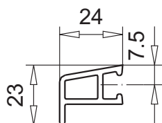
защитная планка арт.№ 109.249 клеммниппель арт.№ 108.016
