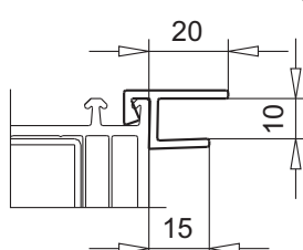
профиль с пазом арт.№ 109.327
