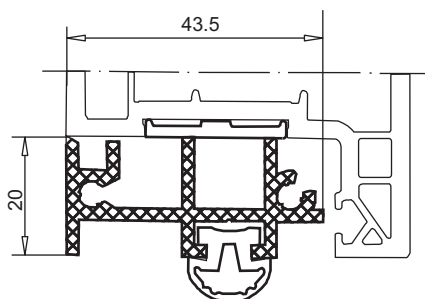
профиль с пазом под уплотнение арт. № 104.010 цвет: белый, коричневый
