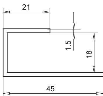
П-образный профиль арт. № 117.833
