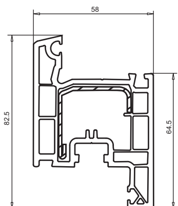
арт. № 103.196 пленка с двух сторон пленка с одной стороны усилитель арт. № 113.306 усилитель арт. № 113.310 (цветное исполнение для окон) усилитель арт. № 113.218.2 (цветное исполнение для дверей)
