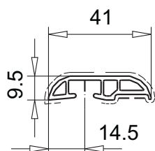
облицовочный профиль арт.№ 109.484 заглушка арт.№ 109.485 Цвет: белый, коричневый клеммниппель арт.№ 108.016
