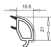
арт. №107.238 контур SWINGLINE
