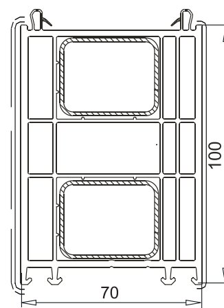
расширитель 100мм арт.№ 114.203 усилитель арт.№ 113.271 усилитель арт.№ 113.271.4
