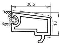
штапик арт. № 107.569
