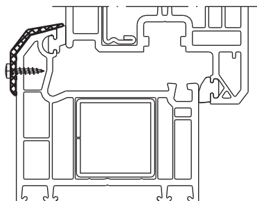
арт. № 104.200 верхняя часть порожка алюминиевый Цвет: E6/EV1, Euras 15
