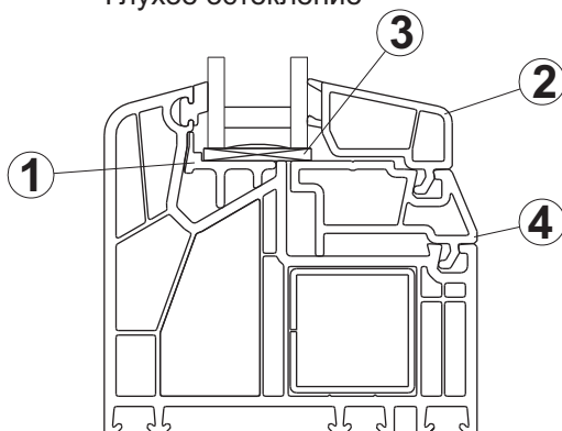
Глухое остекление
