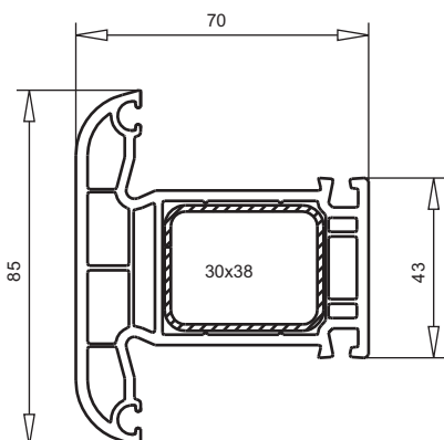
арт. № 102.235 пленка с двух сторон пленка с одной стороны усилитель арт. №113.271 усилитель арт. №113.271.4
