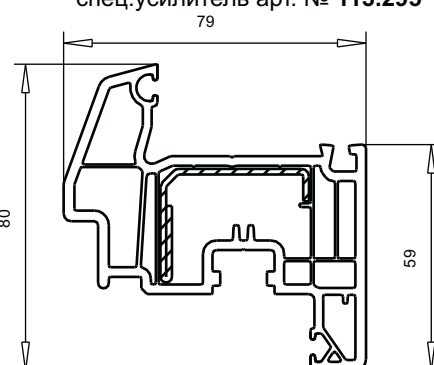
арт. № 103.240
