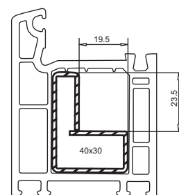
арт. № 113.009 специальный усилитель для ответных частей фурнитуры в рамах 101.085 / 101.111
