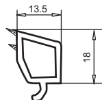
штапик арт. № 107.213 толщина стеклопакета 24+24,5 мм
