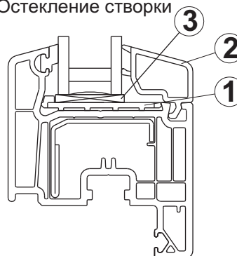
Остекление створки
