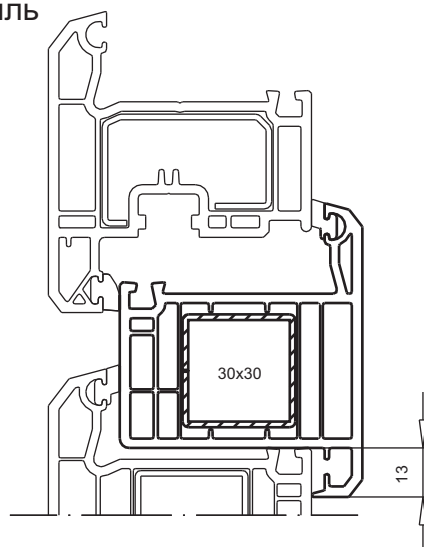
арт. № 102.232 переходной профиль усилитель арт. № 113.271 усилитель арт. № 113.271.4 использовать только в комбинации с импостом арт.№102.200
