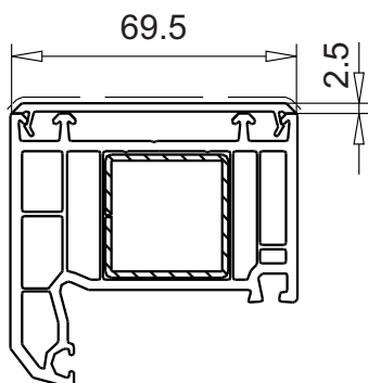
маскирующий профиль арт.№ 109.495
