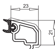
арт. №107.200 контур TOPLINE
