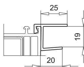
профиль с пазом арт.№ 109.342
