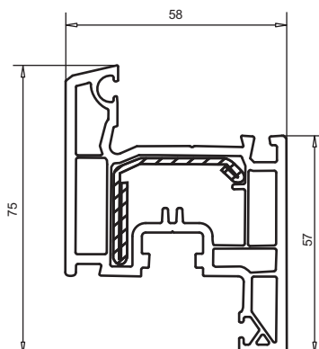
арт. № 103.213 усилитель арт. № 113.229
