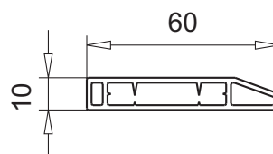
траверса арт.№ 109.014
