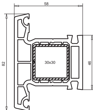
арт. № 102.103 пленка с двух сторон пленка с одной стороны усилитель арт. № 113.025 сварка только в соединении с рамой
