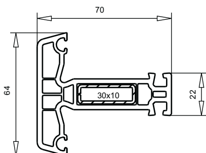
арт. № 102.237 створочная перекладина пленка с двух сторон пленка с одной стороны усилитель ат. № 113.020
