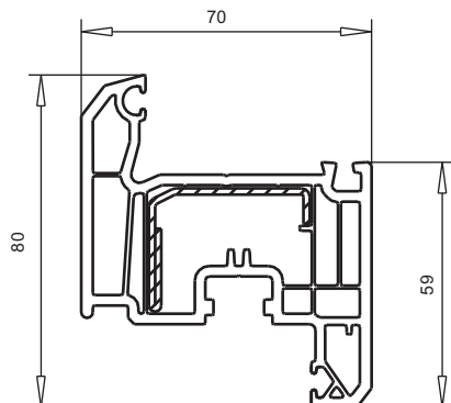
арт. № 103.212 пленка с двух сторон пленка с одной стороны усилитель арт. №113.292 усилитель арт. №113.294 усилитель арт. №113.295
