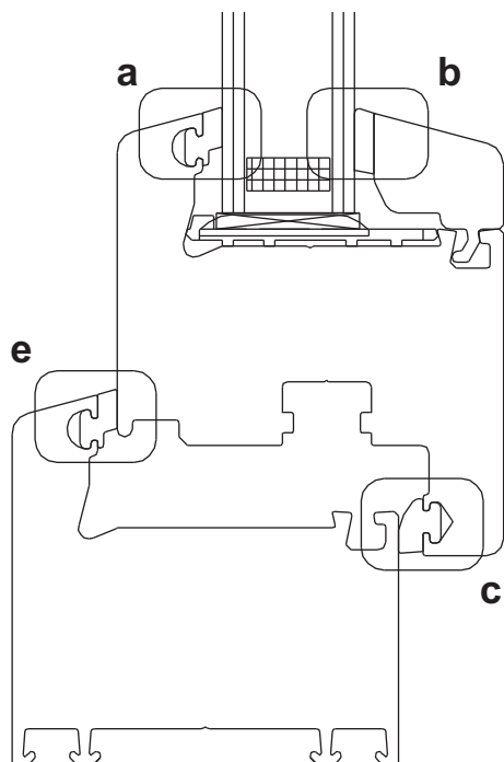
Фальцевое уплотнение
