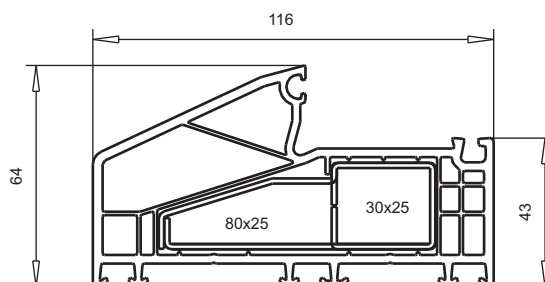
арт. № 101.282 усилитель арт. № 113.002 усилитель арт. № 113.003
