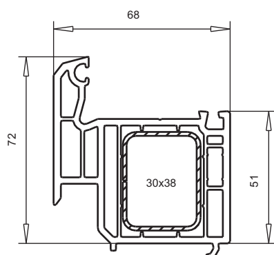
арт. № 103.206 расширительный профиль пленка с двух сторон пленка с одной стороны усилитель арт. № 113.271
