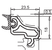
штапик арт. № 107.555
