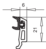
арт. №107.208 контур TOPLINE
