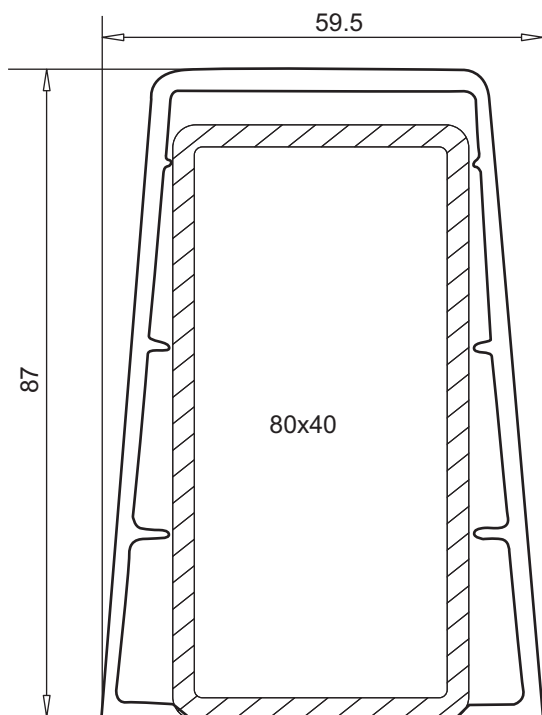
внешний усилитель 59,5x87 мм
