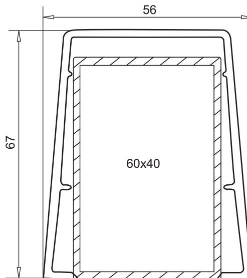
внешний усилитель 56x67 мм
