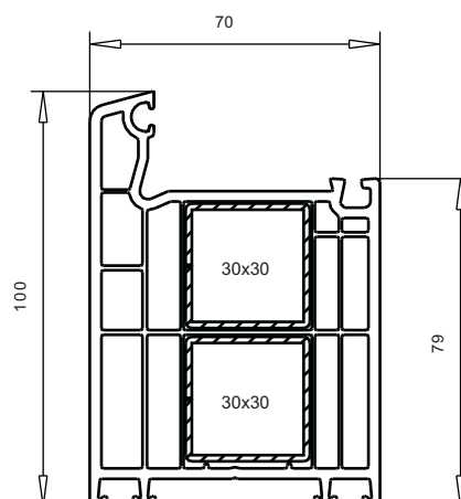
арт. № 101.215 пленка с двух сторон пленка с одной стороны усилитель арт. № 113.025
