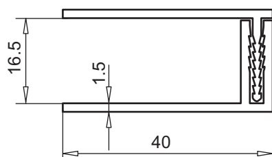
выравнивающий профиль арт. № 117.835
