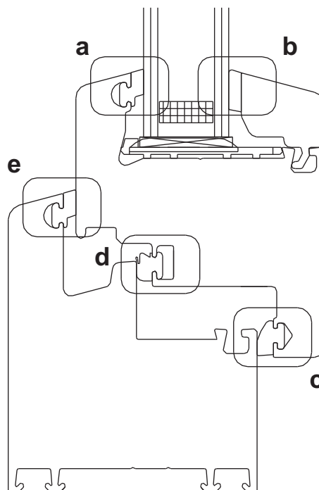
Среднее уплотнение
