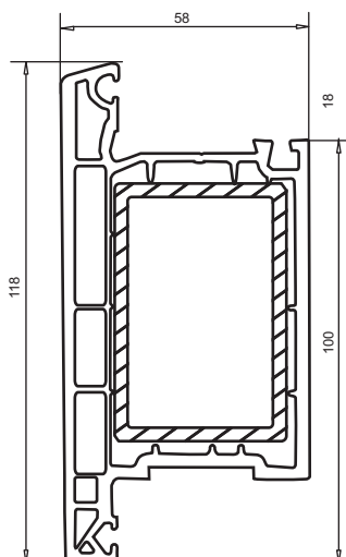
арт. № 105.124 дверная створка открывается наружу пленка с двух сторон пленка с одной стороны усилитель арт. № 113.011.3
