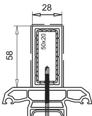
внешний усилитель 28x58мм арт.№ 109.082 усилитель арт.№ 113.047 I_x=1,41\text{см}^4 , I_y=6,21\text{см}^4
