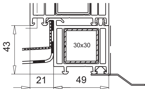
расширительный профиль для балконной двери арт.№ 109.445 усилитель арт.№ 113.025 специальная анкерная пластина арт.№ 141.137
