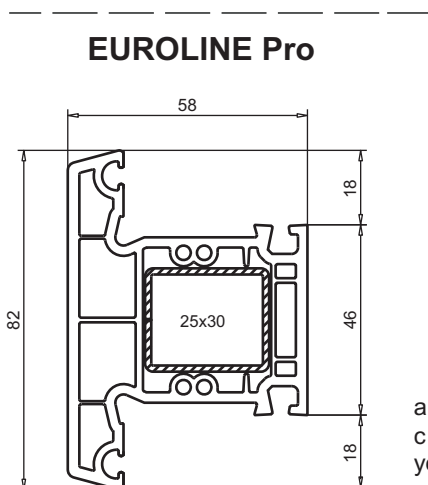
арт. № 102.087 пленка с двух сторон пленка с одной стороны усилитель арт. № 113.025
