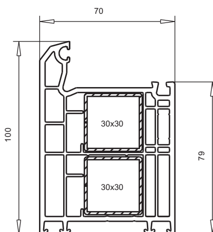
арт. № 101.202 пленка с двух сторон пленка с одной стороны усилитель арт. № 113.025
