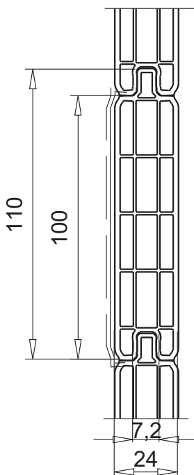
вагонка арт.№ 109.361
