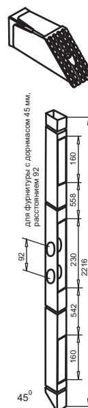
арт. № 113.005.5 60x40x3мм длина 2240 мм
