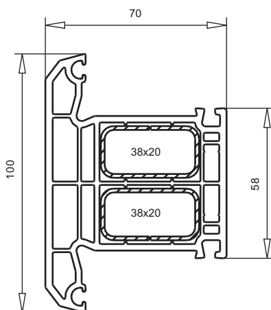
арт. № 102.207 пленка с двух сторон пленка с одной стороны усилитель арт. №113.272
