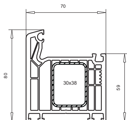
арт. № 101.285 SOFTLINE XXL усилитель арт. № 113.271 усилитель арт. № 113.302
