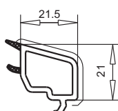
арт. №107.224 контур SOFTLINE
