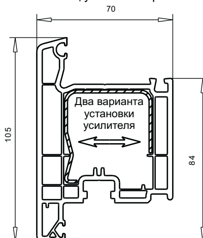
арт. № 103.242
