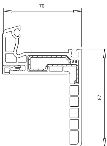
арт. № 111.280 пленка с одной стороны пленка с двух сторон усилитель арт. № 113.212
