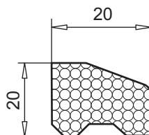
закрывающая планка арт. № 117.810
