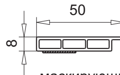
маскирующий профиль 50мм арт.№ 109.443.3 с клеящейся лентой 19х1мм, черный
