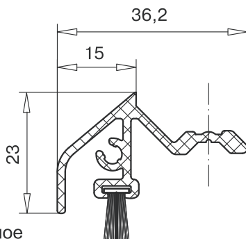
Слезник алюминиевый М 1:1
