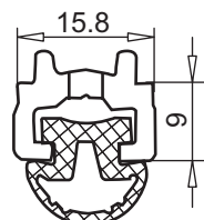
профиль под паз 16 мм для уплотнения арт. № 112.026 арт. № 104.129 для уплотнения входной двери арт. № 112.026 черный полимерный материал перфорир.
