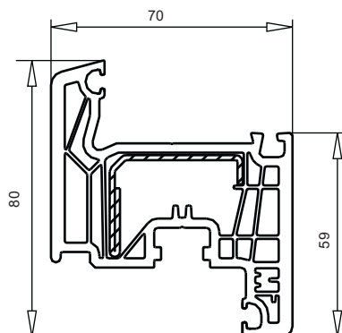
арт. № 103.303 Softline XXL усилитель арт. №113.292 усилитель арт. №113.294 усилитель арт. №113.295
