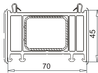
расширитель 45мм арт.№ 114.202 усилитель арт.№ 113.271 усилитель арт.№ 113.271.4
