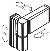
арт. № 140.318 петля VEKA для входной двери из двух частей, для створки весом до 120 kg регулируется в 3 плоскостях, установка с обеих сторон цвет: белый / Euras 15 (коричневый) шаблон арт. № 146.011.7
