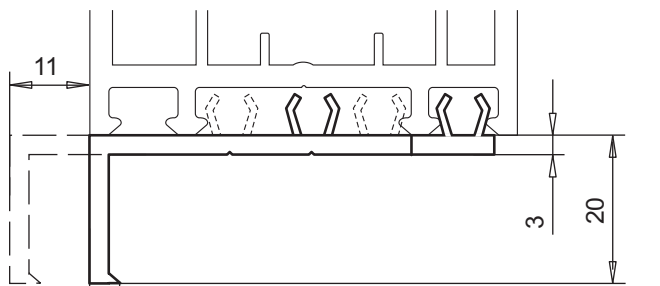
присоединительный профиль арт. № 109.071
