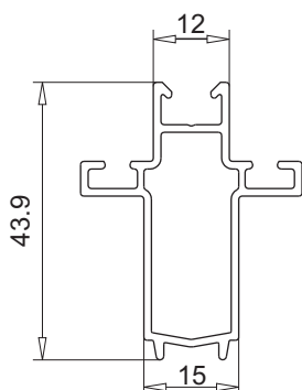
арт. № 105.779 штульп заглушка арт. № 109.650
