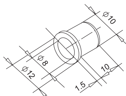
водоотводная трубка арт. № 143.062 цвет: прозрачный наружный диаметр \varnothing 10 мм / общая длина 11.5 мм
