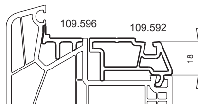
вставка арт. № 109.592 фальцевый вкладыш арт. № 109.596 Цвет: красный
