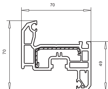
арт. № 103.201 пленка с двух сторон пленка с одной стороны усилитель арт. №113.269
