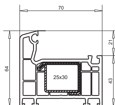
арт. № 101.286 усилитель арт. № 113.010 усилитель арт. № 113.002
