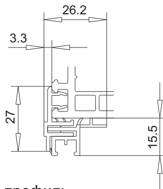
маскирующий профиль арт. № 109.480/109.481
