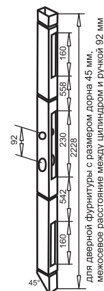
арт. № 113.286.5 65x45x43 мм 2228 мм длина
