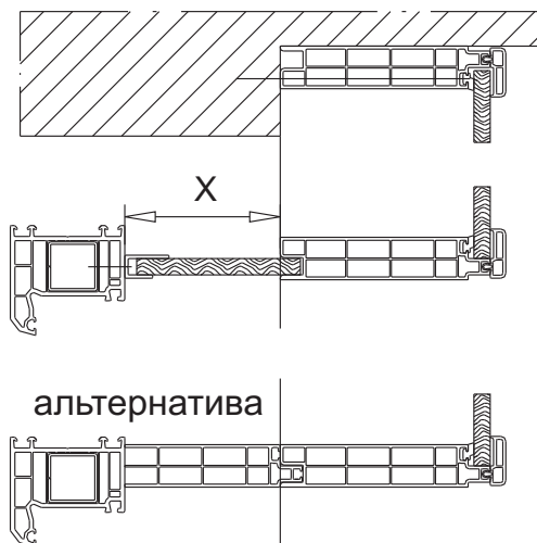
Сечение А
