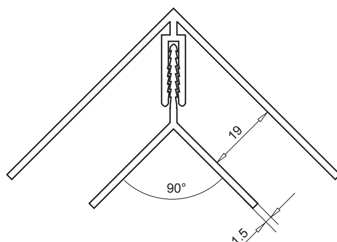
уголок арт. № 117.836
