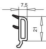
арт. №107.228 контур SWINGLINE
