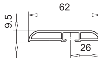
облицовочный профиль арт.№ 109.499 заглушка арт.№ 109.500 Цвет: белый клеммниппель арт.№ 108.016
