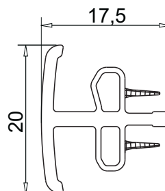
соединитель с уплотнением арт. № 116.217
