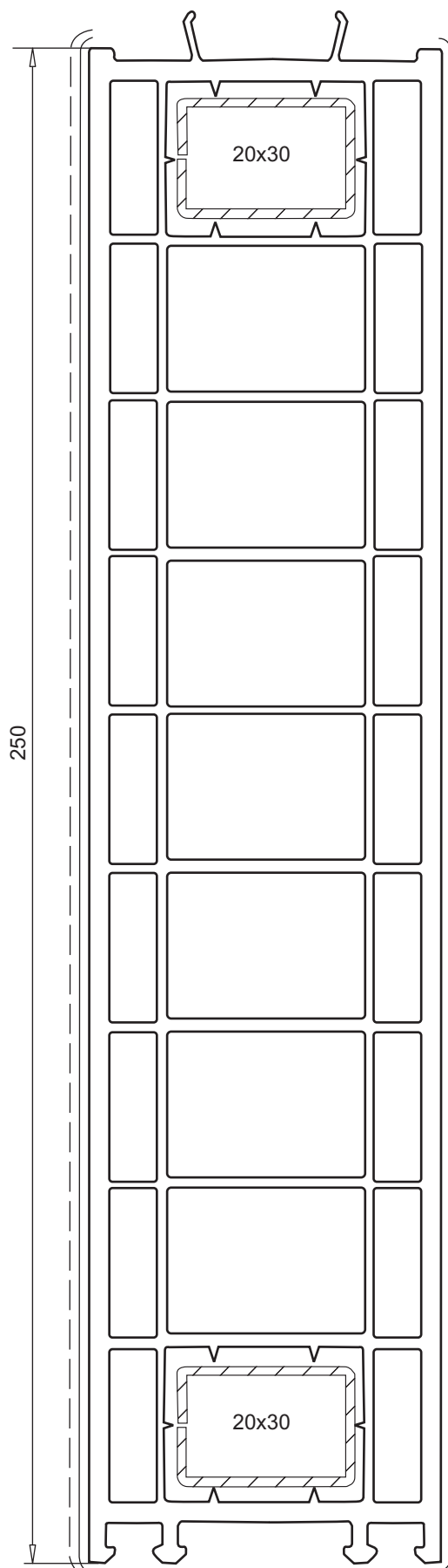
расширитель 250 мм арт. № 114.005 усилитель арт. № 113.019
