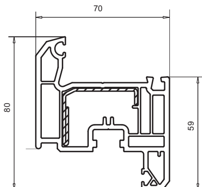
арт. № 103.200 усилитель арт. № 113.292
