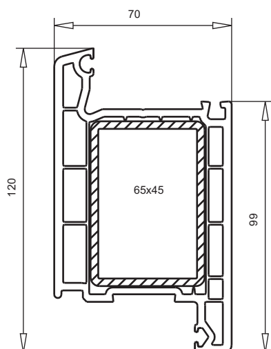
арт. № 105.232 дверная створка пленка с двух сторон пленка с одной стороны усилитель арт. № 113.286.3 алюмин.усилитель арт. № 115.200
