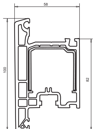
арт. № 103.219 дверная створка открывается наружу пленка с двух сторон пленка с одной стороны усилитель арт. № 113.049.2 усилитель арт. № 113.147.2
