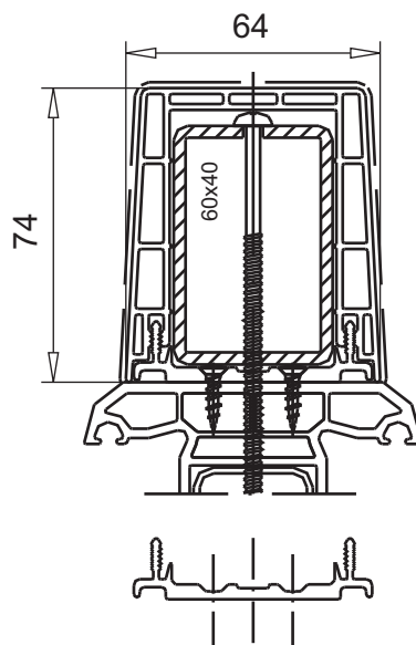
внешний усилитель 64x74мм арт.№ 114.031 усилитель арт.№113.011.2 I_x=10,23\text{см}^4 , I_y=19,31\text{см}^4 усилитель арт.№113.011.3 I_x=14,32\text{см}^4 , I_y=27,39\text{см}^4
