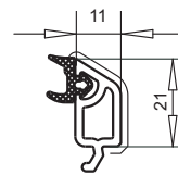
арт. №107.220 контур SOFTLINE
