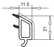
арт. №107.218 контур SOFTLINE
