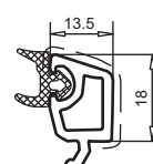
штапик арт. № 107.582
