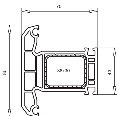
арт. № 102.200 пленка с двух сторон пленка с одной стороны усилитель арт. №113.271 усилитель арт. №113.271.4
