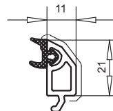
арт. №107.204 контур TOPLINE
