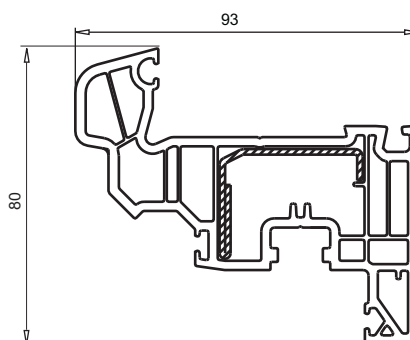
арт. № 103.315 , псм пленка с двух сторон пленка с одной стороны усилитель арт. №113.292 усилитель арт. №113.294 усилитель арт. №113.295
