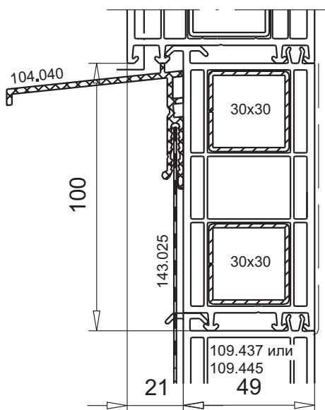
расширительный профиль для балконной двери арт.№ 109.437 усилитель арт.№ 113.025 (2x) специальная анкерная пластина арт.№ 141.137
