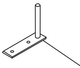
соединительный профиль арт. № 116.012 основа белого цвета \Rightarrow белое уплотнение основа коричневого цвета \Rightarrow черное уплотнение усилитель арт. № 113.061 I_x=58,60 \text{ см}^4 , усилитель арт. № 113.061.1 I_x=8,17 \text{ см}^4 монтажная пластина арт. № 141.433
