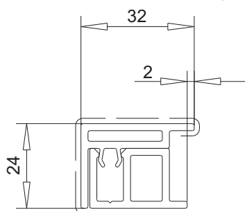
маскирующий профиль арт. № 109.184/109.185
