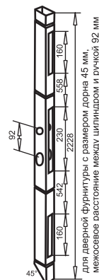
арт. № 113.286.5 65x45x43 мм 2228 мм длина
