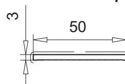
полоса 50мм арт.№ 109.052
