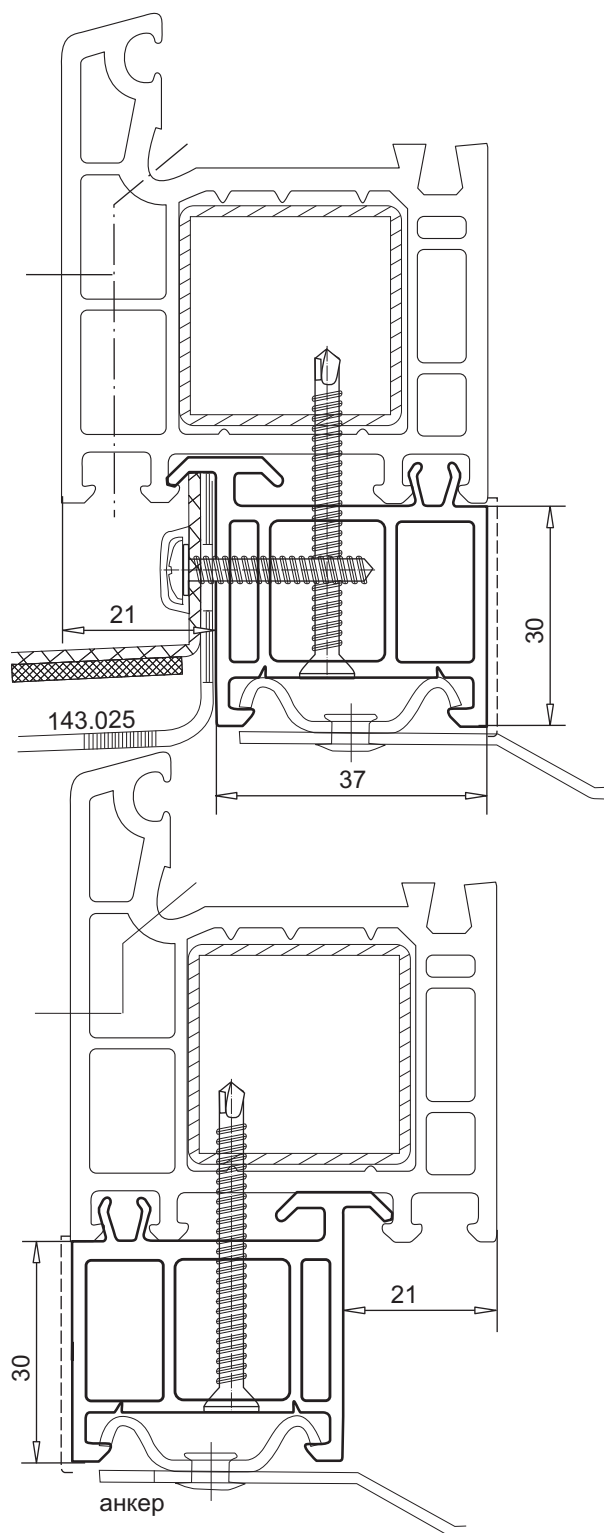
профиль для присоединения балконной двери 30 мм арт. № 109.304
