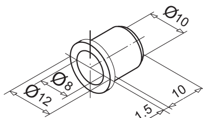
набегающая подкладка арт. № 109.203 цвет белый
