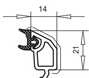
арт. №107.203 контур TOPLINE
