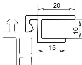
П-образный профиль арт. № 109.254
