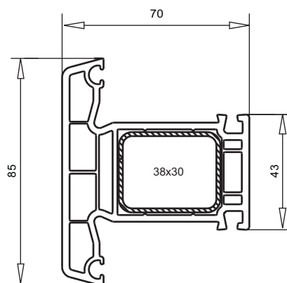
арт. № 102.218 пленка с двух сторон пленка с одной стороны усилитель арт. № 113.271 усилитель арт. № 113.271.4
