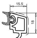
штапик арт. № 107.570
