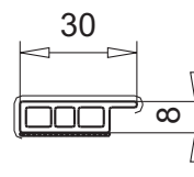
только со стороны помещения маскирующий профиль арт.№ 109.166.2 с черной клеящейся лентой
