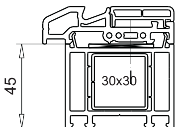
арт. № 114.011 расширитель усилитель арт. № 113.025
