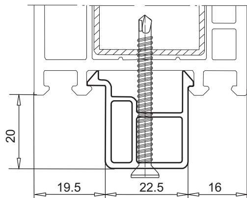
защитный профиль арт. № 110.001 второсырье
