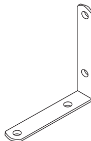
соединительный уголок арт. № 141.400.7 83,5/83,5/20 мм
