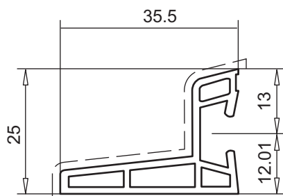
конечная планка арт. № 109.419
