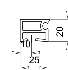
маскирующий профиль арт.№ 109.020 клеммниппель арт.№ 108.016
