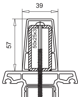
внешний усилитель арт.№ 114.018 усилитель 50x25x3.0 арт.№ 113.161.3 I_x=3.99\text{см}^4 ; I_y=12.55\text{см}^4
