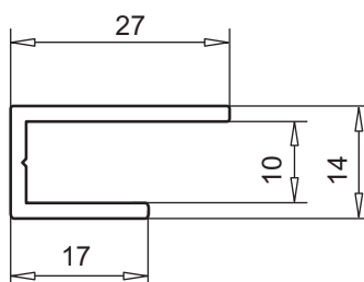
П-образный профиль арт. № 109.254
