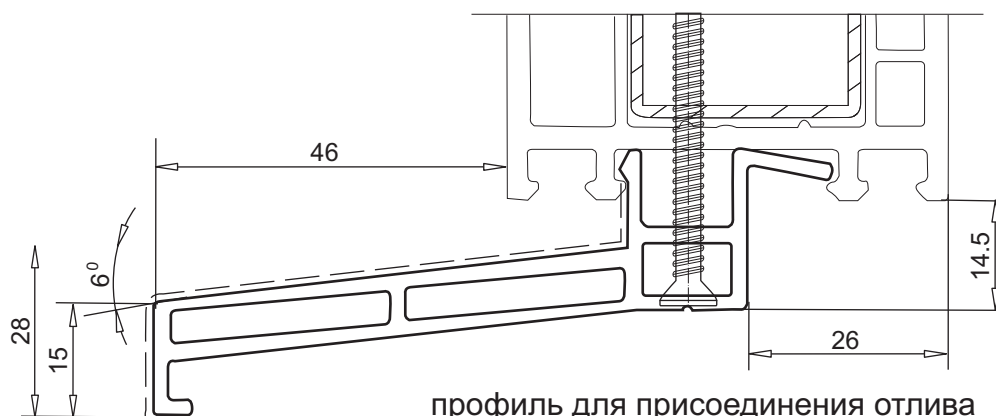
профиль для присоединения отлива арт. № 110.028
