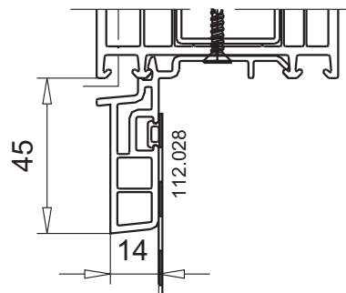
подставочный профиль арт.№ 110.111
