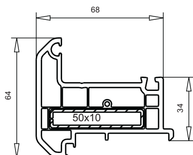
арт. № 102.215 пленка с двух сторон пленка с одной стороны усилитель арт. № 113.013 усилитель арт. № 113.013.3 (стальная пластинка)
