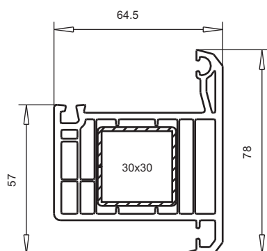
арт. № 102.229 усилитель арт. № 113.025
