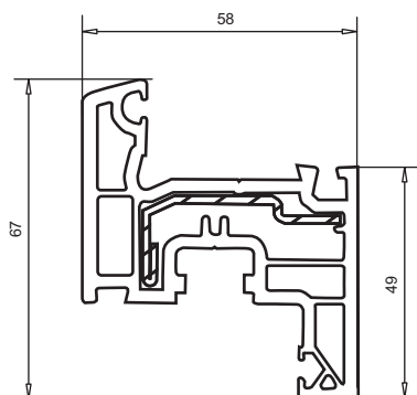
арт. № 103.214 пленка с двух сторон пленка с одной стороны усилитель арт. № 113.091
