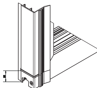
Длина закрывающей планки: высота створки - 2 x 25 мм Две заглушки снизу и сверху
