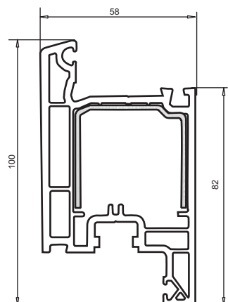
арт. № 103.198 дверная створка открывается внутрь пленка с двух сторон пленка с одной стороны усилитель арт. № 113.049.2 усилитель арт. № 113.147.2
