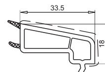
штапик арт. № 107.130
