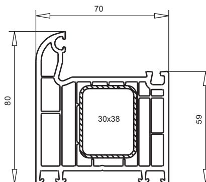
арт. № 101.235 пленка с двух сторон пленка с одной стороны усилитель арт. №113.025
