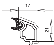
арт. №107.202 контур TOPLINE
