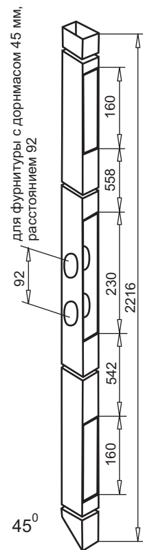
арт. № 113.005.5 60x40x3 мм длина 2240 мм
