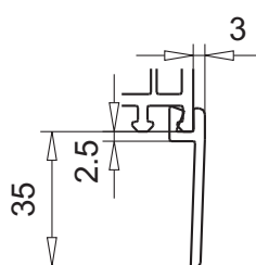
облицовочный профиль арт.№ 109.402 клипсовое соединение на раму, только с внутренней стороны
