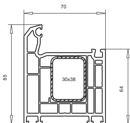
арт. № 101.203 пленка с двух сторон пленка с одной стороны усилитель арт. № 113.271
