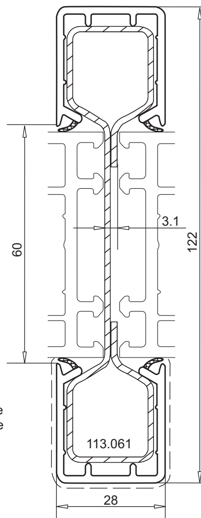
соединительный профиль арт. № 116.012 основа белого цвета \Rightarrow белое уплотнение основа коричневого цвета \Rightarrow черное уплотнение усилитель арт. № 113.061 I_x=58,60 \text{ см}^4 , усилитель арт. № 113.061.1 I_x=8,17 \text{ см}^4 монтажная пластина арт. № 141.433
