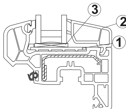
Остекление створки
