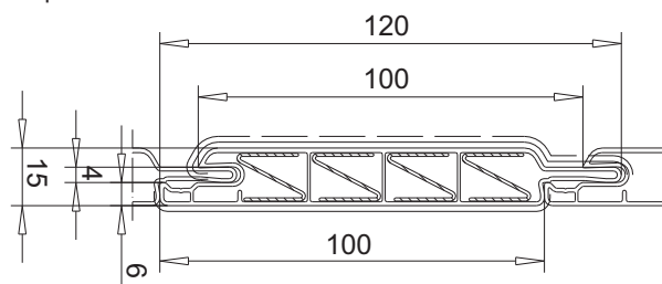
маскирующий профиль арт. № 109.020
