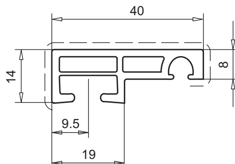
облицовочный профиль арт. № 109.104
