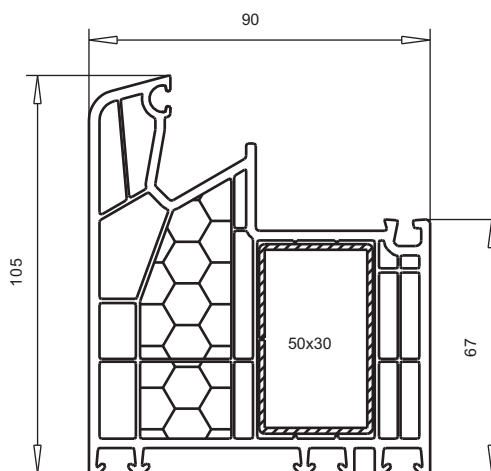
арт. № 101.237 пленка с двух сторон пленка с одной стороны усилитель арт. №113.046
