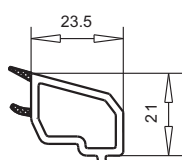
арт. №107.244 контур TOPLINE
