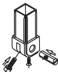
арт. № 141.313 соединитель с изменяемым углом в наборе - соединитель - поперечный штырь - винт с вн. шестигранником - пружинные шайбы - шуруп M4x11
