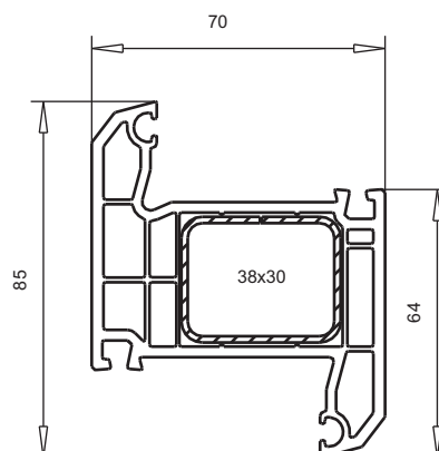
арт. № 102.232 переходной профиль усилитель арт. № 113.271 усилитель арт. № 113.271.4 использовать только в комбинации с импостом арт.№102.200
