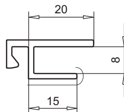
стыкующий профиль арт. № 109.286
