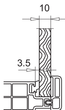
планка арт.№ 109.583
