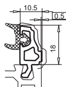
штапик арт. № 107.594
