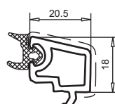
штапик арт. № 107.567
