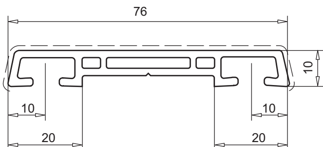
облицовочный профиль арт. № 109.208
