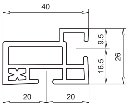
присоединительный профиль арт. № 109.073
