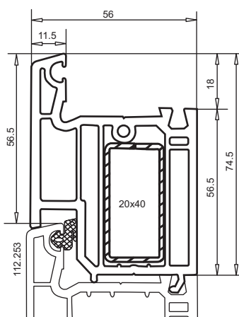
арт. № 103.138 расширительный профиль усилитель арт. № 113.004 уплотнение арт. № 112.253
