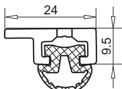
профиль под паз 24 мм для уплотнения арт. № 112.026 арт. № 104.128 для уплотнения входной двери арт. № 112.026 черный полимерный материал с клейкой лентой перфорир.
