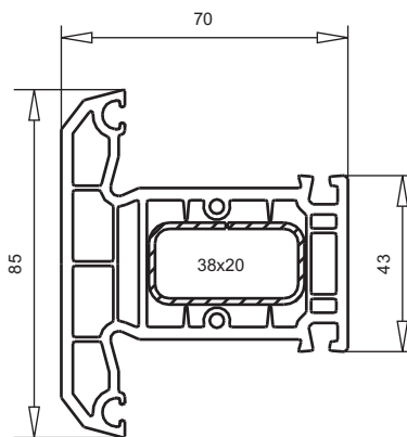
арт. № 102.239 пленка с двух сторон пленка с одной стороны усилитель арт. №113.272
