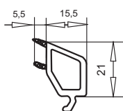
арт. №107.217 контур SOFTLINE
