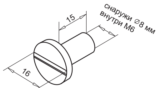
гильза для SL арт. № 141.124.2 никелированная латунь
