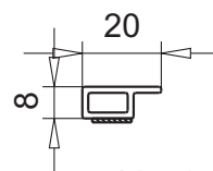
маскирующий профиль 20мм арт.№ 109.442.3 с клеящейся лентой 10х1мм, черный
