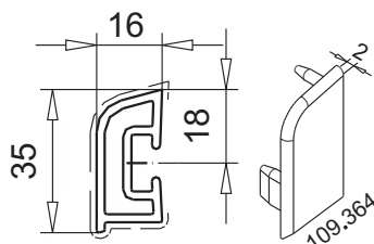
защитная планка арт.№ 109.347 заглушка арт.№ 109.364 Цвет: белый, коричневый, охра, черный клеммниппель арт.№ 108.016
