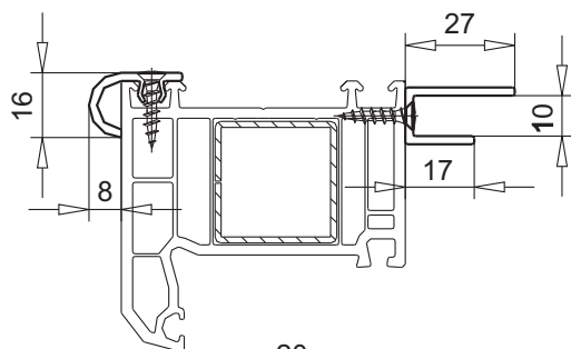
скругляющий профиль арт.№ 108.100
