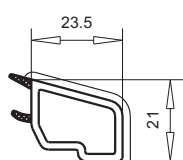
арт. №107.214 контур SOFTLINE
