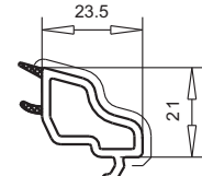
арт. №107.226 контур SOFTLINE
