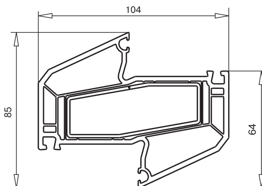
арт. № 102.231 переходной профиль усилитель арт. №113.331/113.343.2
