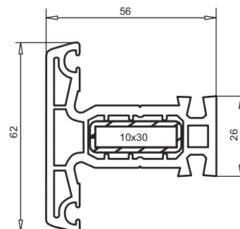
арт. № 102.084 пленка с двух сторон пленка с одной стороны усилитель арт. № 113.020
