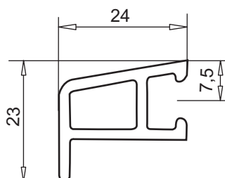
маскирующий профиль арт. № 109.249
