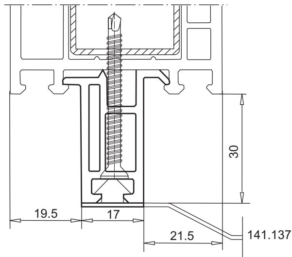
профиль для присоединения отлива арт. № 110.053 анкер с захватом 141.137
