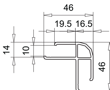
облицовочный профиль арт.№ 109.208 клеммниппель арт.№ 108.016
