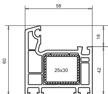
арт. № 101.287 усилитель арт. № 113.002 усилитель арт. № 113.060
