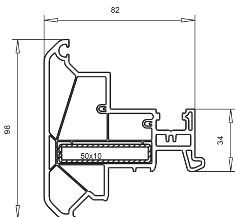
арт. № 102.245 пленка с двух сторон пленка с одной стороны усилитель арт. №113.013 усилитель арт. №113.013.3
