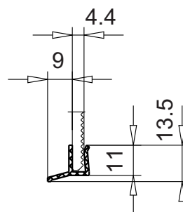
алюмин.планка арт.№ 109.080 для 111.007 / 016 / 024 цвет: алюмин.красный, Euras 15 (коричневый элоксированный)
