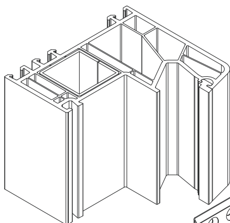
арт. № 104.270 порог ПВХ серый
