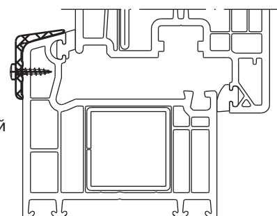
арт. № 104.107 защита рамы от истирания 25x17,5 мм алюмин. E6/EV1, Euras 15, белый
